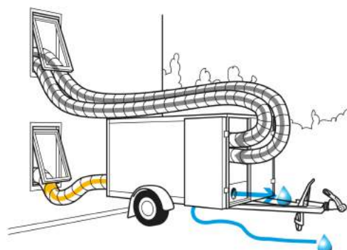
Beispiel Außenaufstellung
